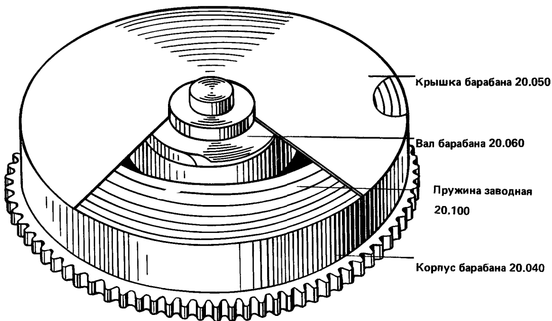
Барaban с валом и пружиной 20.010
