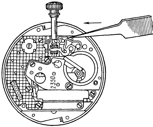
Рис. 117. Установка вала переводного в механизм Установить вал переводной в механизм и вернуть рычаг переводной в исходное положение.
