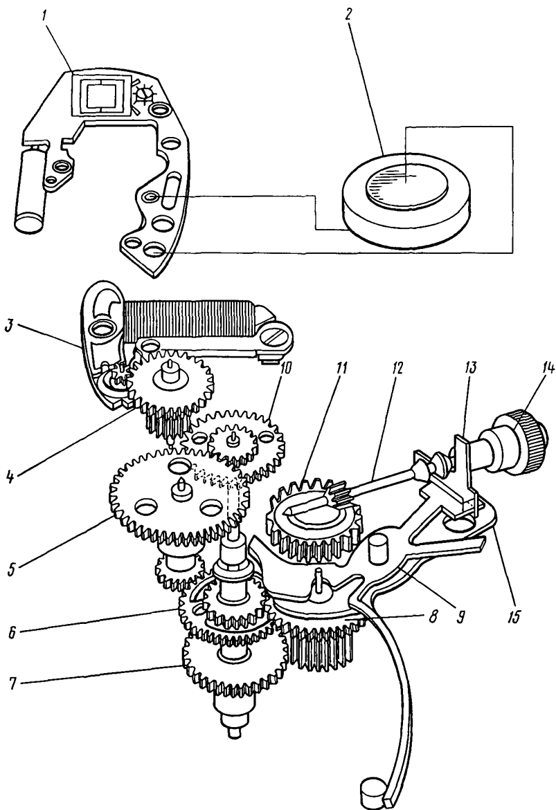
Рис. 4. Кинематическая схема механизма часов 1656А: 1 – блок кварцевого генератора; 2 – источник питания; 3 – шаговый двигатель; 4 – колесо передаточное; 5 – колесо промежуточное; 6 – колесо центральное; 7 – колесо часовое; 8 – колесо минутное; 9 – рычаг обнуления; 10 – колесо секундное; 11 – колесо переводное; 12 – вал переводной; 13 – пластина; 14 – головка переводная; 15 – рычаг переключения
