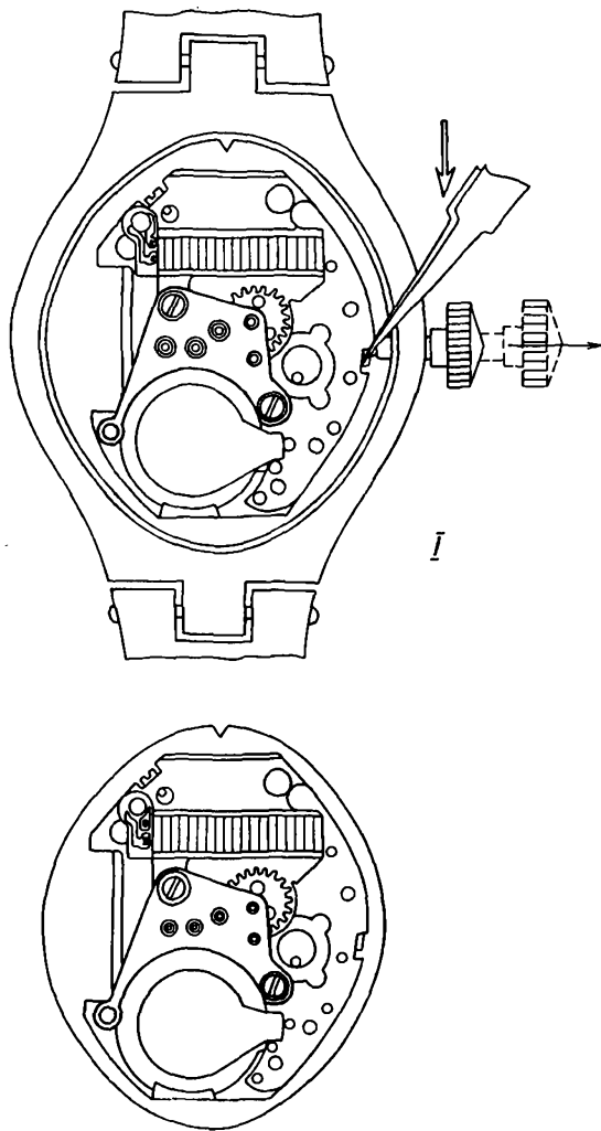
Рис. 22. Извлечение механизма из корпуса: I – для извлечения механизма из корпуса необходимо вынуть из механизма вал переводной, отодвинув пластину концом пинцета или отвертки
