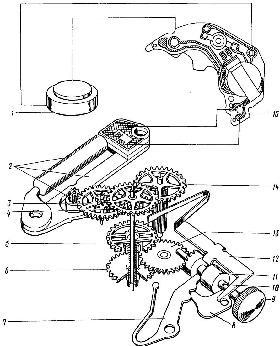
Рис. 5. Кинематическая схема механизма часов 1656Н:
