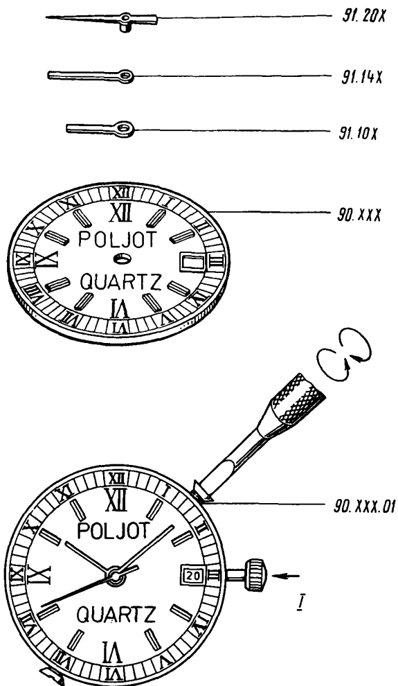
Рис. 159 90.XXX – циферблат; 90.XXX.01. – винт циферблата; 91.10X – стрелка часовая; 91.14X – стрелка минутная; 91.20X – стрелка секундная; I – установить вал переводной в механизм Примечание: отвернуть винты крепления циферблата на 1,5–2 оборота и после снятия циферблата довернуть винты до упора
