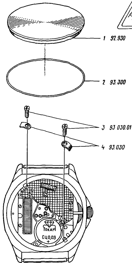
Рис. 140 1 – крышка (дно); 2 – прокладка корпуса; 3 – винт скобы крепления; 4 – скоба крепления
