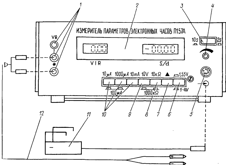
Рис. 15. Расположение органов управления прибора П157А: 1 – входные гнезда „VR“, „I“ и „*“; 2 – цифровое табло; 3 – переключатель интервала времени измерения хода часов; 4 – ручка регулировки усиления сигнала; 5 – разъем для подключения индукционного датчика; 6 – переключатель напряжения встроенного источника питания; 7 – кнопка контроля встроенного источника питания; 8 – кнопка диапазона измерения сопротивления; 9 – кнопка диапазона измерения напряжения; 10 – кнопка диапазона измерения тока; 11 – индукционный датчик; 12 – шнур соединительный
