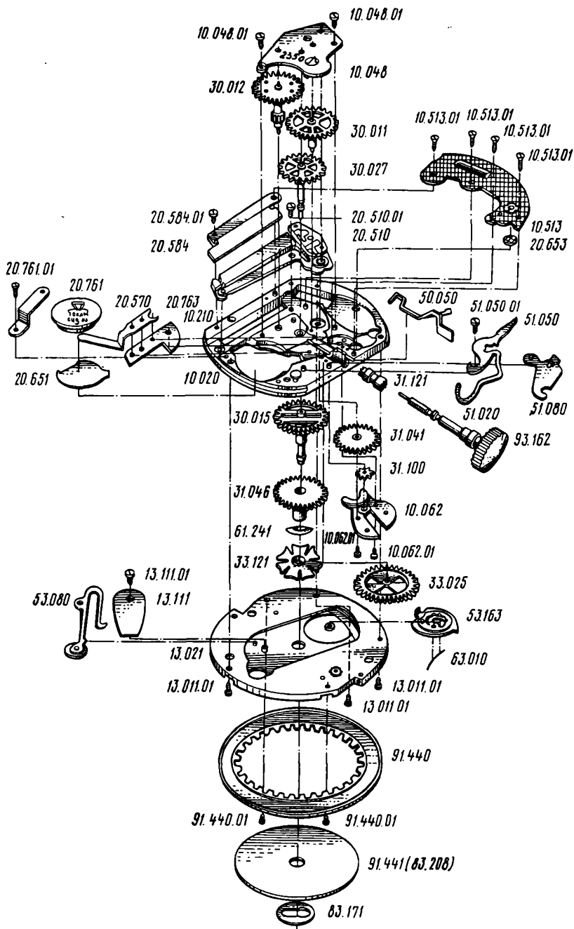
Рис. 113. Детали и сборочные единицы механизма часов 2350, 2360: 10.020 – платина; 10.048 – мост колесной передачи; 10.048.01 – винт моста колесной передачи; 10.062 – мост колеса минутного; 10.062.01 – винт моста колеса минутного; 10.210 – накладка; 10.513 – блок кварцевого генератора; 10.513.01 – винт блока кварцевого генератора; 13.011.01 – винт блока календаря; 13.021 – платина календаря; 13.111 – пластина фиксатора чисел месяца; 13.111.01 – винт пла-
