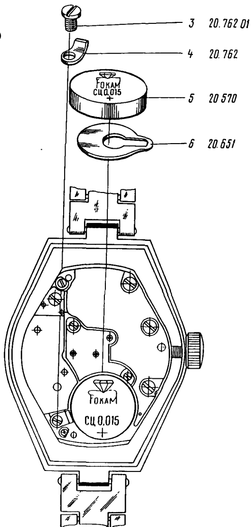
Рис. 93 Примечание: источник питания брать только пластмассовым пинцетом или пинцетом с изолированными концами.
