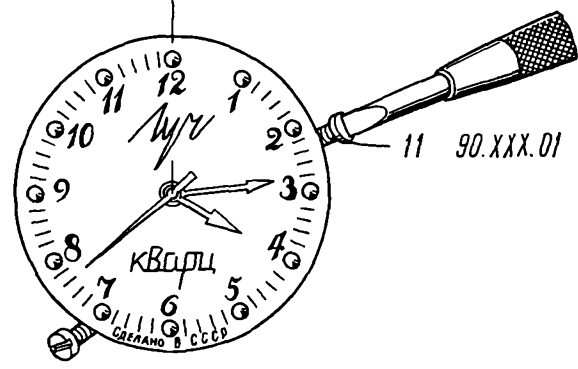
Рис. 50 8 – стрелка секундная; 9 – стрелка минутная; 10 – стрелка часовая; 11 – винты циферблата; 12 – циферблат Примечание: винты крепления циферблата отвернуть на 1,5–2 оборота и после снятия циферблата довернуть винты до упора.
