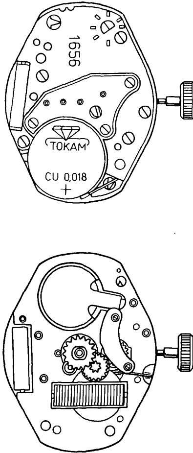
Рис. 44. Механизм часов 1656
