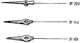
Рис. 134 90.XXX – циферблат; 90.XXX.01 – винт циферблата; 91.10X – стрелка часовая; 91.14X – стрелка минутная; 91.20X – стрелка секундная.
