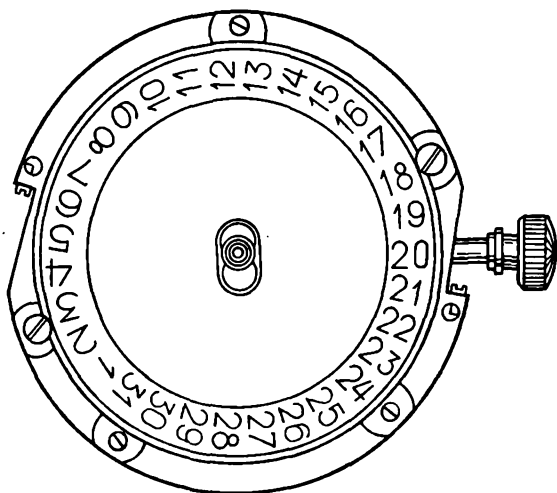
Рис. 133. Механизм часов 2360
