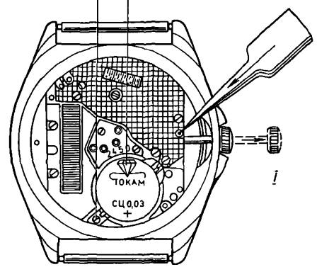
Рис. 141 I – вынуть из механизма вал переводной, нажав на ось рычага переводного концом пинцета Примечание: источник питания брать пластмассовым пинцетом или пинцетом с изолированными концами.
