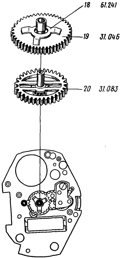
Рис. 70 Примечание: фольга с колеса часового не снимается.
