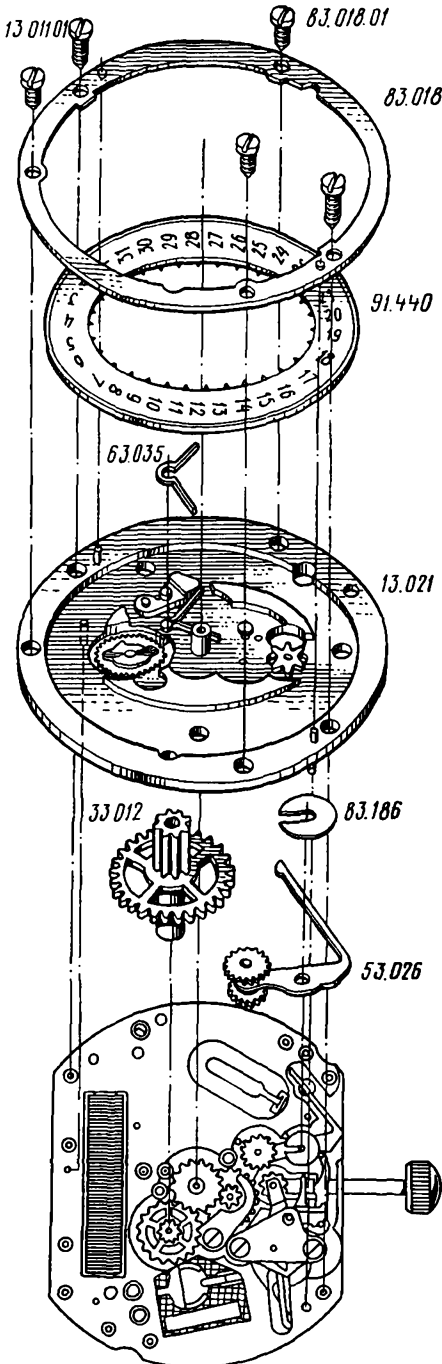
Рис. 157. Детали и сборочные единицы календарного устройства механизма часов 2460:
