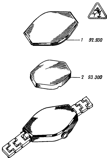
Рис. 92 1 – крышка (дно); 2 – прокладка корпуса (кожух)
