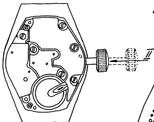
Рис. 94. Извлечение механизма из корпуса: I – для извлечения механизма из корпуса необходимо вынуть из механизма вал переводной, нажав на ось рычага переводного концом пинцета или отвертки; II – установить вал переводной в механизм
