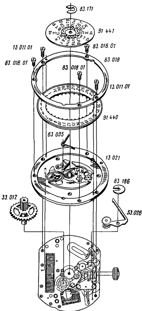
Рис. 139 Детали и сборочные единицы календарного устройства механизма часов 2450:
