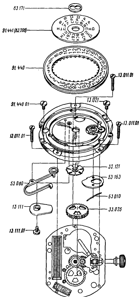
Рис. 114. Детали и сборочные единицы календарного устройства механизма часов 2350, 2360:
