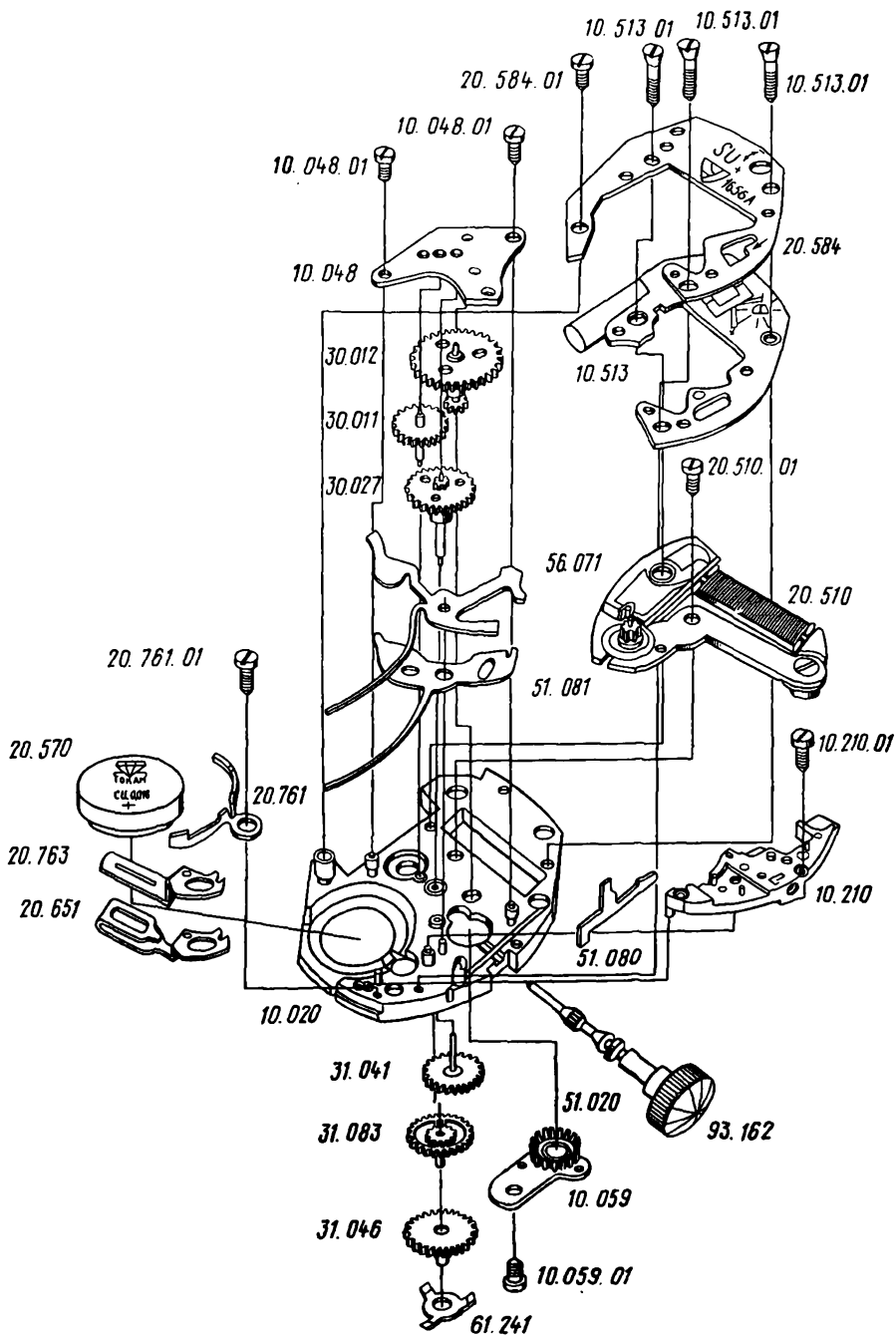
Рис. 65. Детали и сборочные единицы механизма 1656А: 10.020 – платина; 10.048 – мост колесной передачи; 10.048.01 – винт моста колесной передачи; 10.059 – мост колеса переводного; 10.059.01 – винт моста колеса переводного; 10.210 – на-
