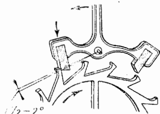
Фиг. 31. Правильный угол притяжки не больше 2°.
