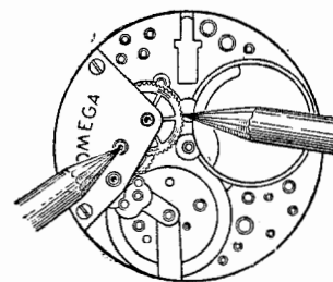
Фиг. 81. Способ проверки глубины зацепления.
