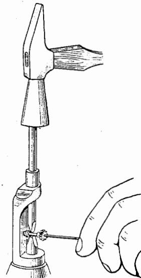
Фиг. 322. Приспособление для создания выступов на минутном трибе.
