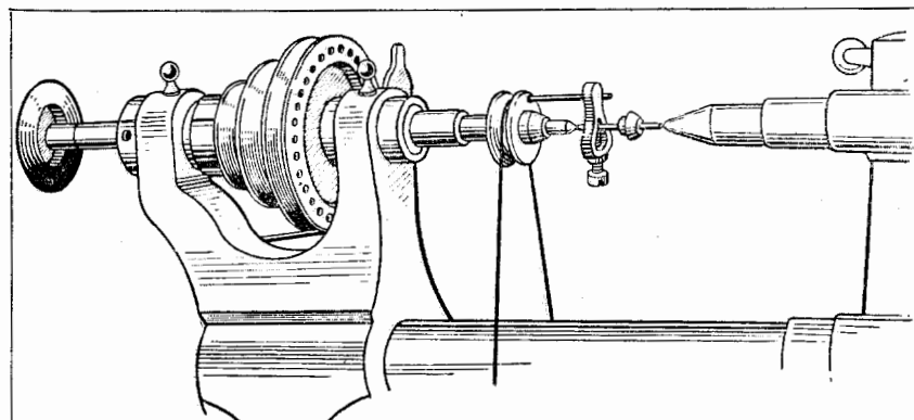
Фиг. 297. Ось баланса, закрепленная в центрах.
