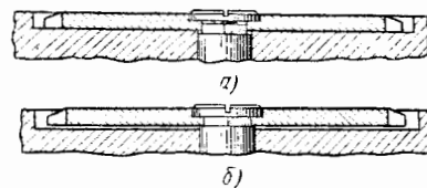
Фиг. 139. Заедание барабанного колеса. Заплекник вала не проходит через платину; a — заклинивание; б — свободное перемещение.
