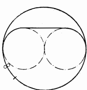
Фиг. 172. Построение концевой кривой для спирали, предназначенной для замены плоской спирали. (Диаметр окружностей, обозначенных пунктирной линией, должен равняться радиусу спирали.)
