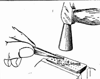
Фиг. 64. Установка нового штифта.
