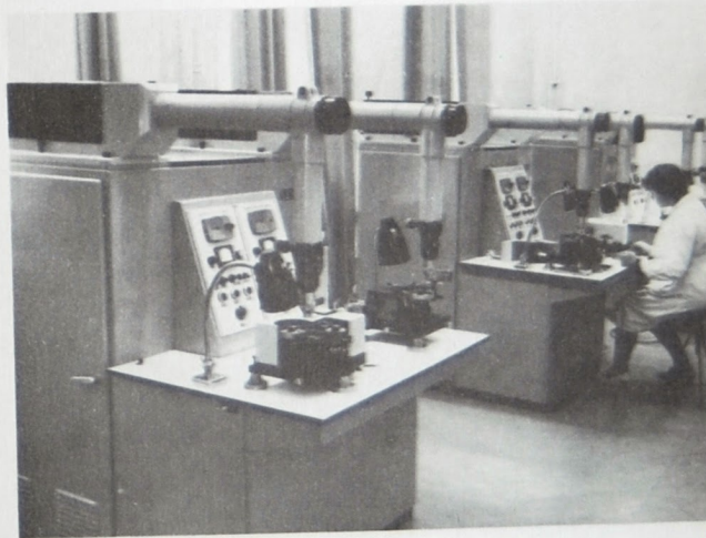
Лазерные установки для прошивки отверстий в часовых камнях.
