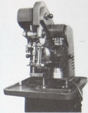
Автомат 3-306 для полировки профиля зубьев мелко модульных часовых трибов методом обката.
