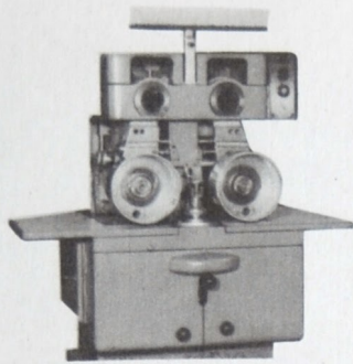
Полуавтомат Ф-328 для алмазной обработки наружных поверхностей часовых корпусов.
